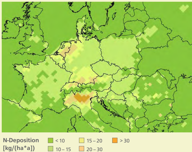
Abbildung 4: Modellerte Stickstoffeinträge in Europa im Jahr 2010 Datenquelle: Buitjes et al. 2011
