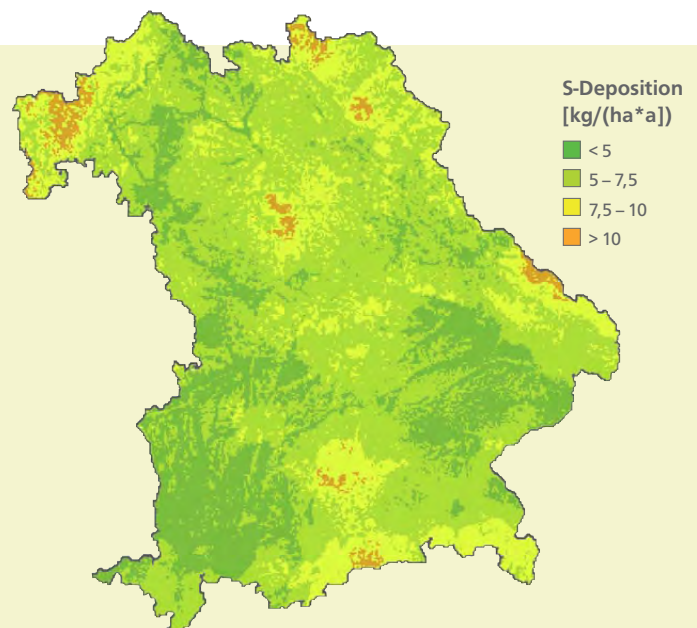
Abbildung 2: Modellierter Schwefeleinträge in Bayern 2007 Datenquelle: Gauger et al. 2008
