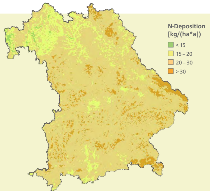
Abbildung 5: Modellerte Stickstoffeinträge in Bayern Datenquelle: Gauger et al. 2008
